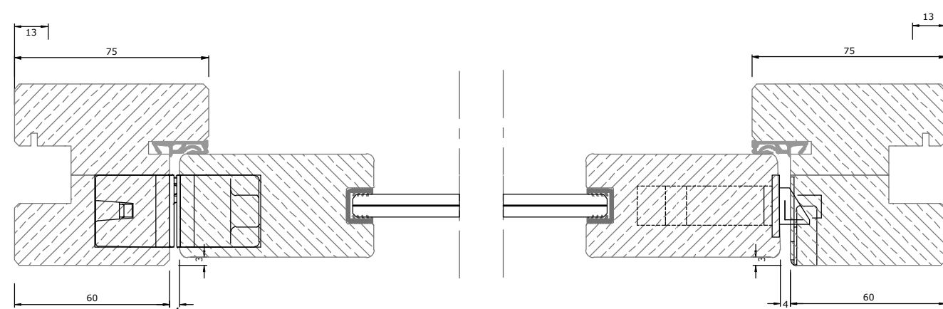
Kaderdeur enkel glas
